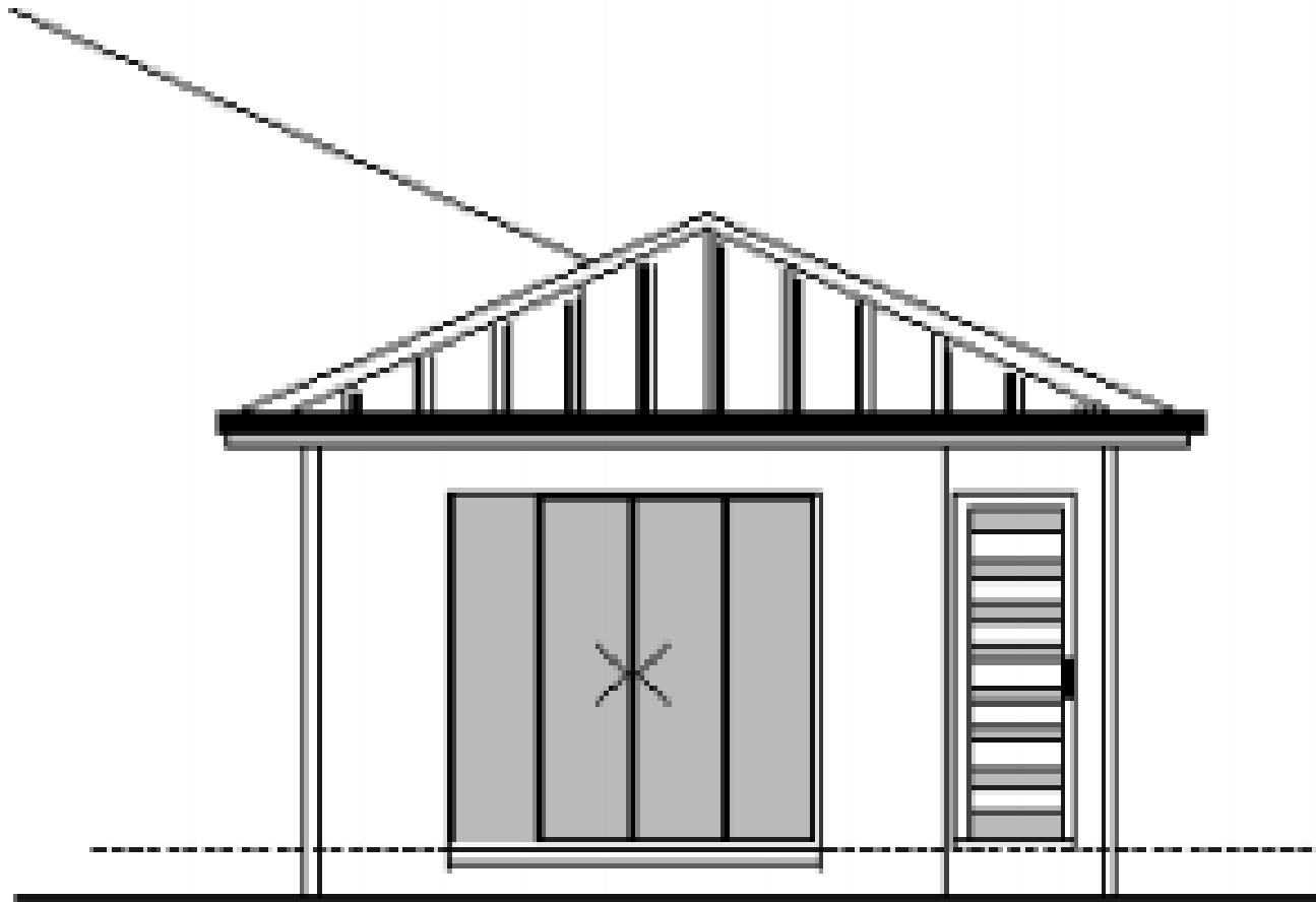
ELEVATION 1
