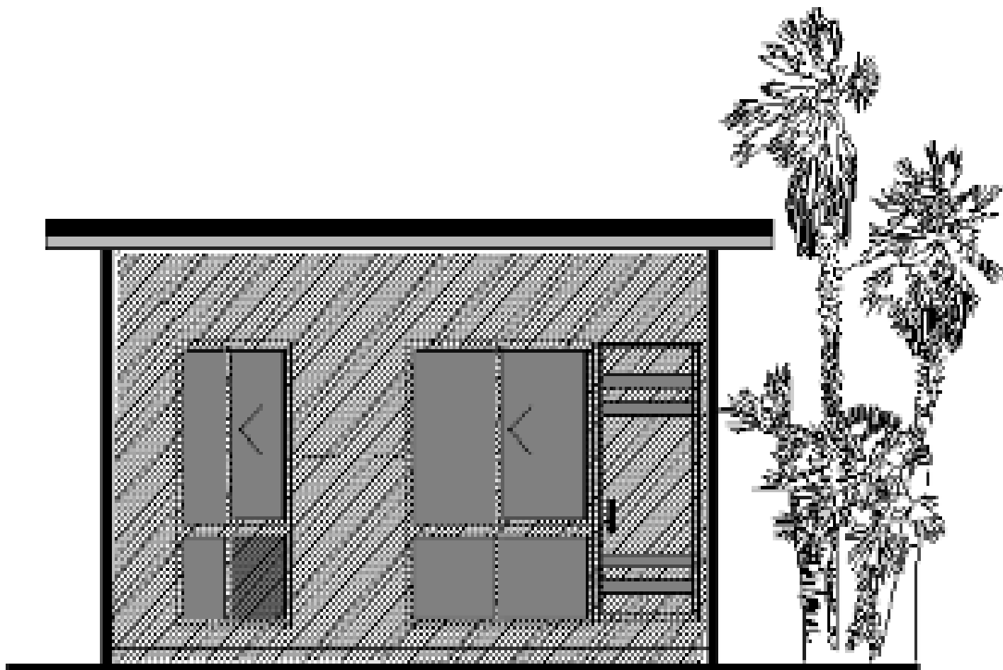
ELEVATION 1
